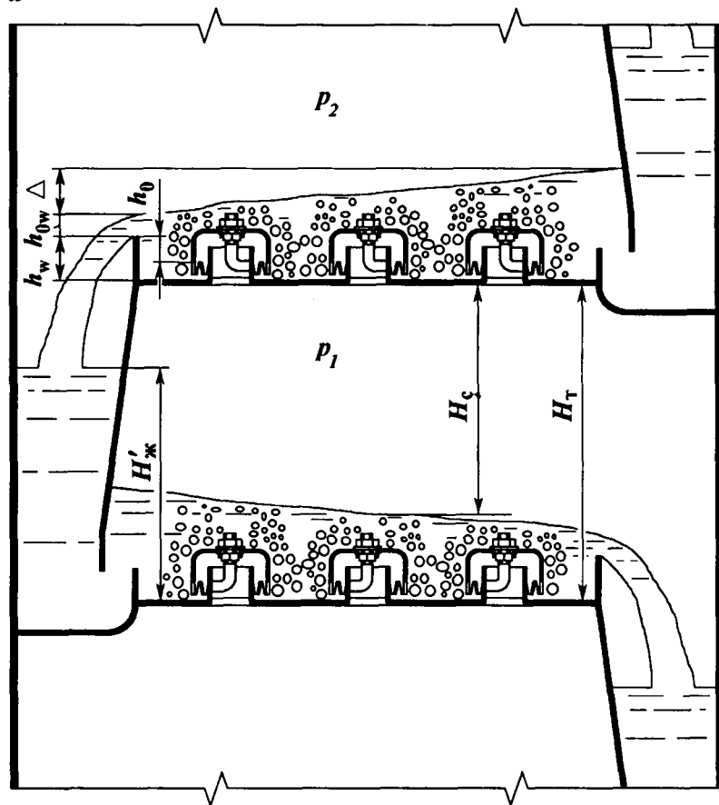
Рис. VII-7. Схема работы барботажной тарелки с круглыми колпачками: a – общий вид тарелки; б – схема барботажга газа в зоне контакта
